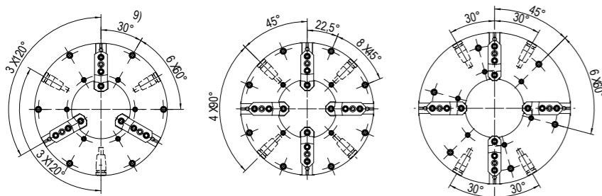
Size 700-1250
