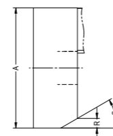
DIN 55029 with studs for Camlock
