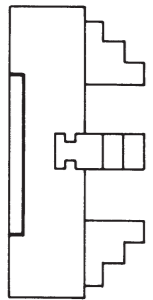
A26 ISO 702-3 (DIN 55027), DIN 55022, with studs and locknuts, optional DIN 55021 with set screw and nut
