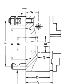
DIN 55027 with studs and nuts
