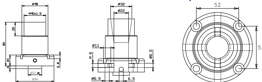
ER32 voor Ø 2-20 mm en NIEUW: Ø 20,5-25 mm (OVERSIZE)
