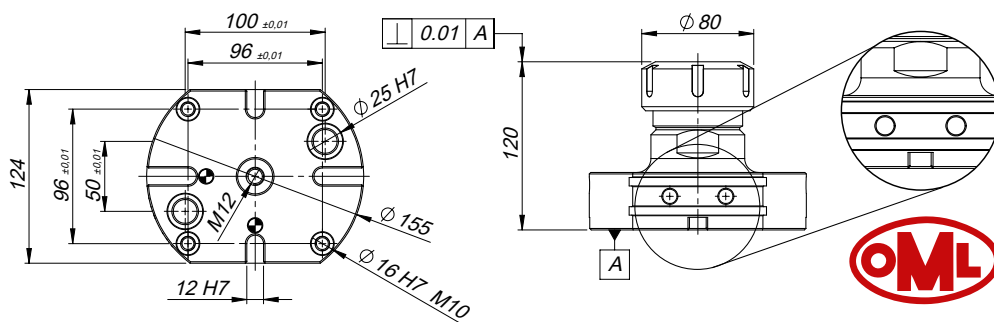
ER50 voor Ø 6-34 mm
