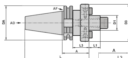
SK50 DIN69871AD
