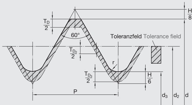
Abb. 1: Bolzengewinde mit Grundmaß 0 (Toleranzlage h) Male thread with basic dimension 0 (tolerance class h)
