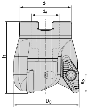
Aufsteckfräser 90° / VC.. 22 Face milling cutter 90° / VC.. 22
